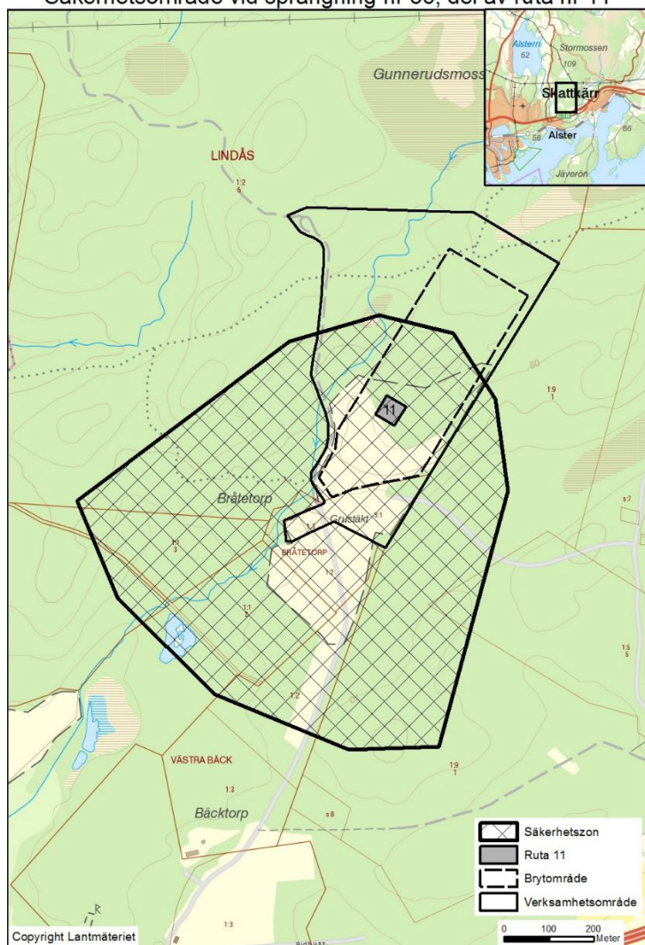
Säkerhetsområde vid sprängning nr 36, del av ruta nr 11
